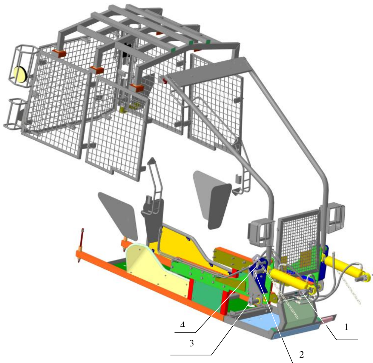
Рисунок 2. Толкатель лесозаготовительный ТЛЗ-1,8.000
