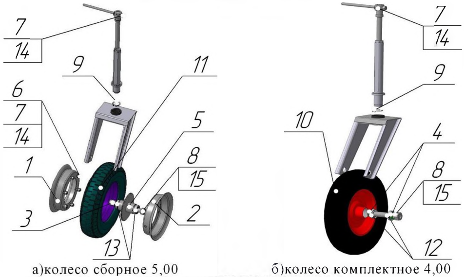
Рисунок 5. Колесо УМДУ-80/82.02.06
