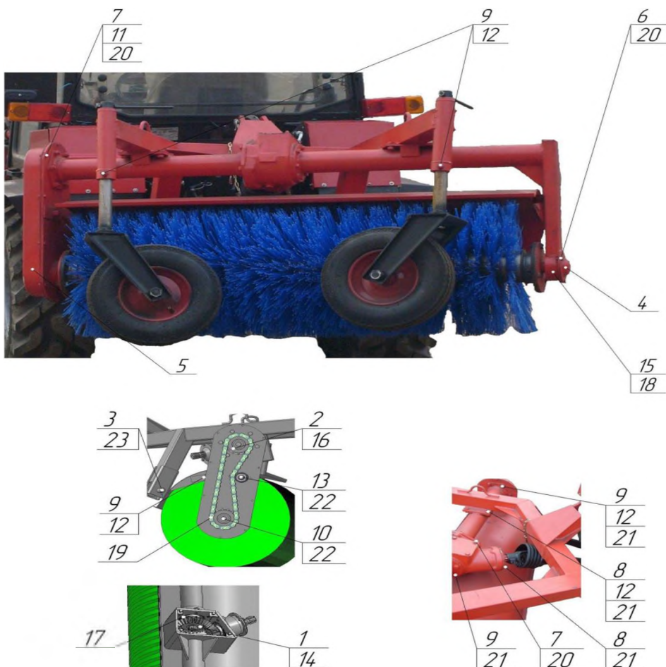
Рисунок 8. Оборудование щеточное УН-320.02
