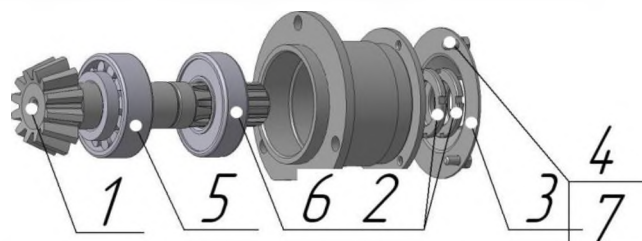
Рисунок 3. Узел ведущей шестерни УМДУ-80/82.02.04
