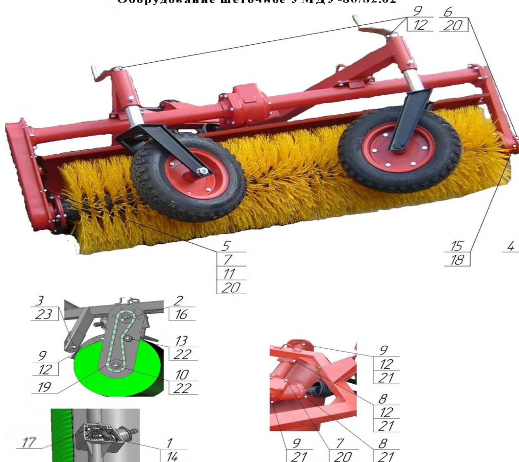
Рисунок 8. Оборудование щеточное УМДУ-80/82.02
