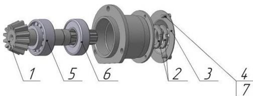
Рисунок 3. Узел ведущей шестерни УМДУ-80/82.02.04
