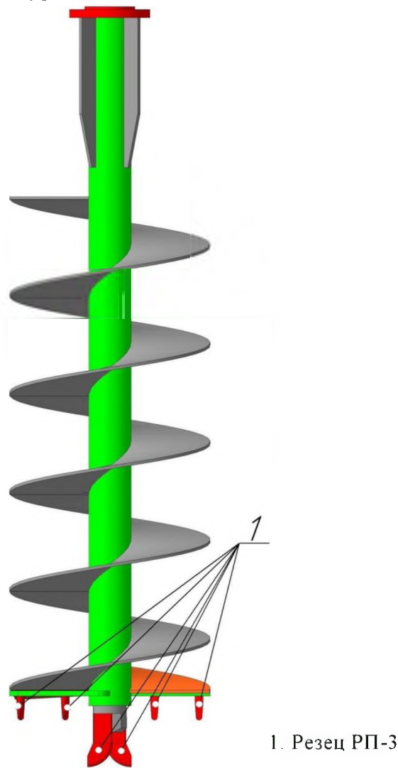
Рисунок 5. Бур НБУ-1300.42
