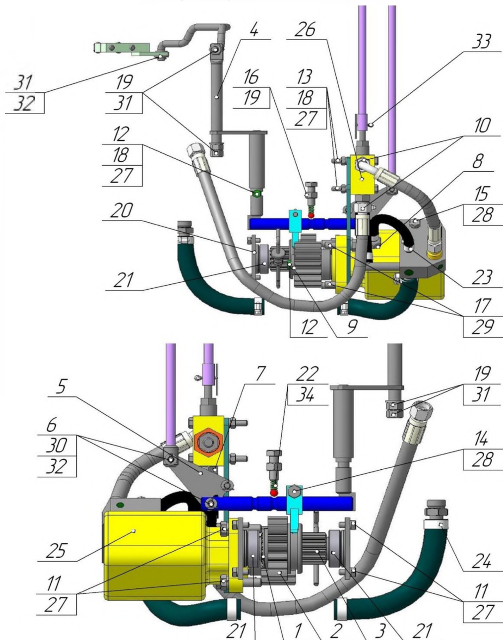
Рисунок 39. Гидроходоуменьшитель ФД-567.11
