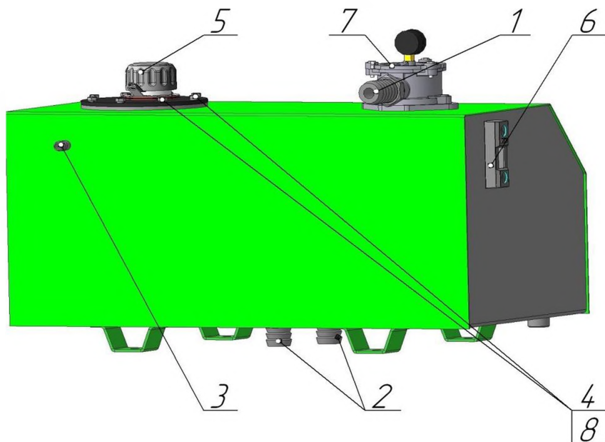
Рисунок 29. Гидробак ШРС-2.02.10
