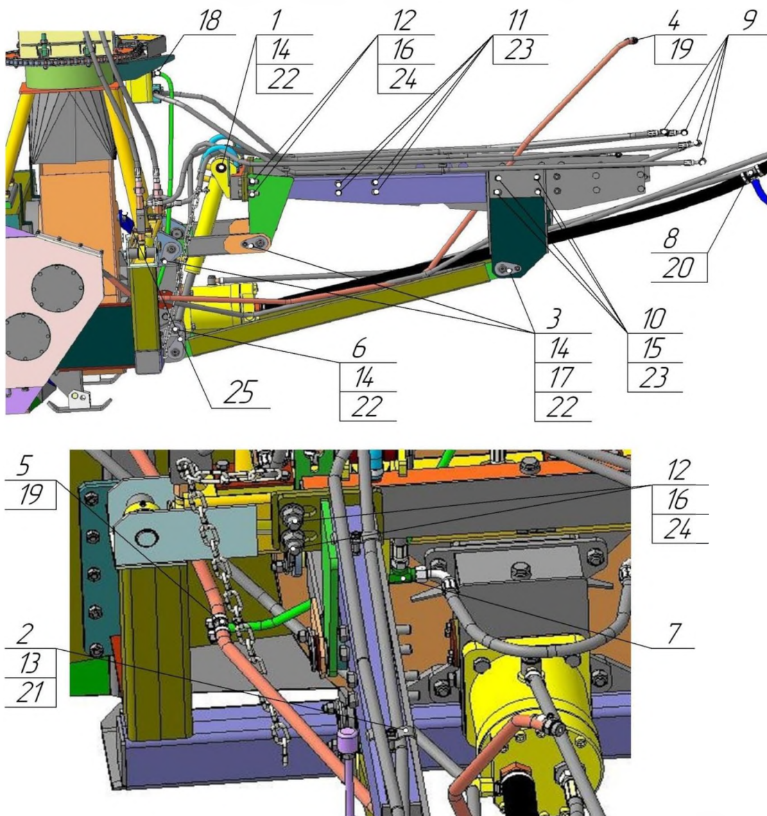
Рисунок 41. Оборудование шнекороторное снегоуборочное ШРК-2,00 с гидравлическим поворотом желоба (с механическим поворотом желоба)
