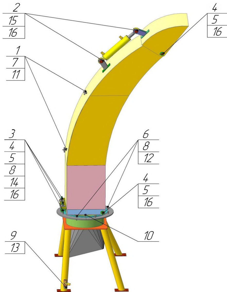
Рисунок 15. Желоб погружочный ШРС-2.01.08-01 (с механическим поворотом желоба)
