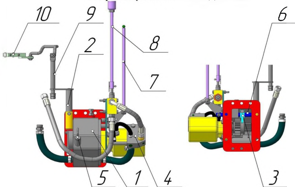
Гидроходоуменьшитель ФД-567.11
