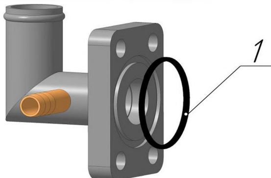
Рисунок 24. Фланец подачи ШРС-2.02.30
