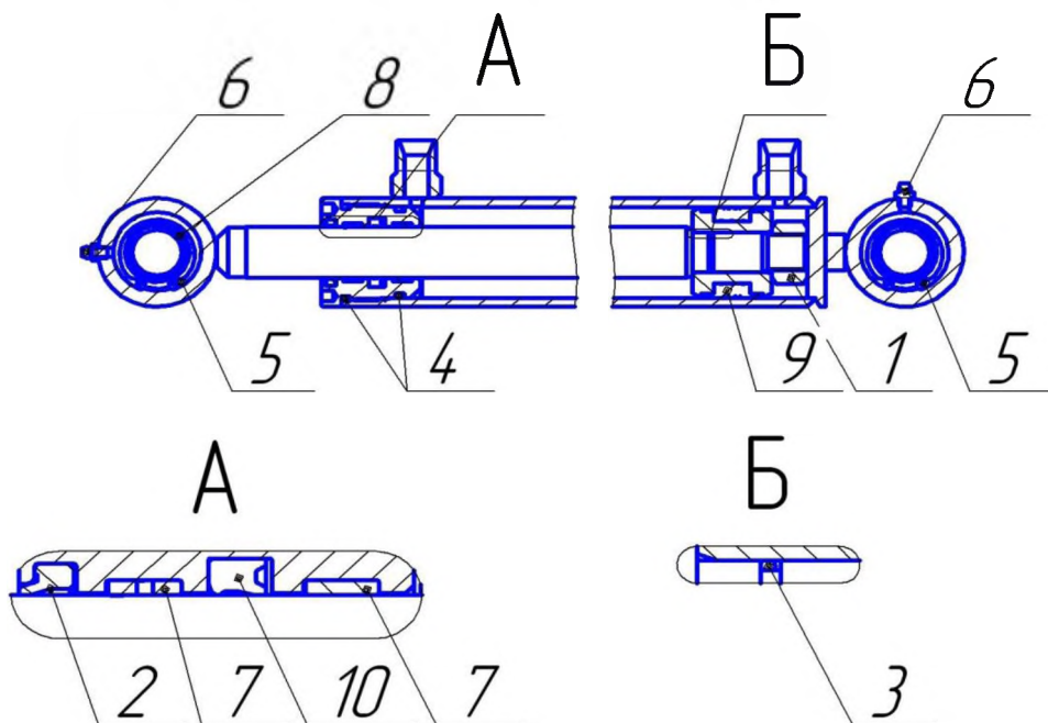
Рисунок 18. Гидроцилиндр ЦГ-ПМК-50.28.440.680-Е1-Р15
